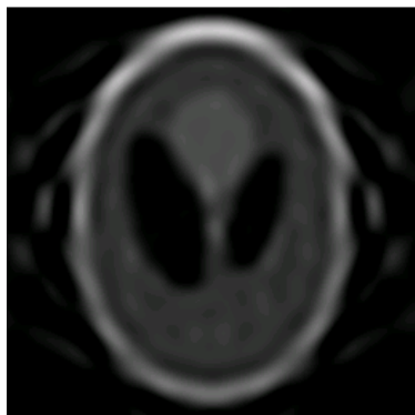
I_{fan1}
