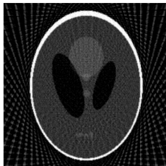
I2
