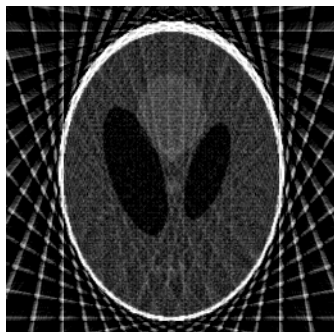
I1
